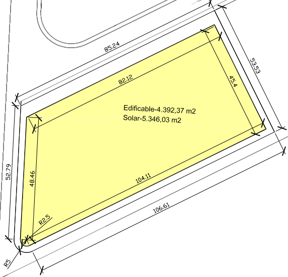
SITUACIÓN PARCELA " PALMA SECTOR 3 INDUSTRIAL " Escala: 1/1.500
